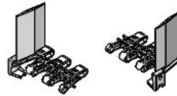
DS5214A - LH 75MM MSG DS5234A - RH 75MM MSG
